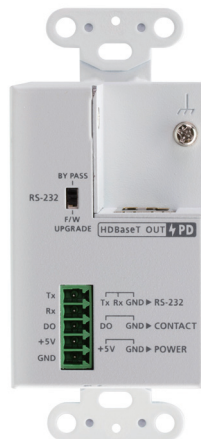
VE1801AUST 후면부
