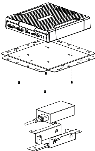
KE6948A DNV 壁掛板與電源變壓器固定架 (2K-0011)
