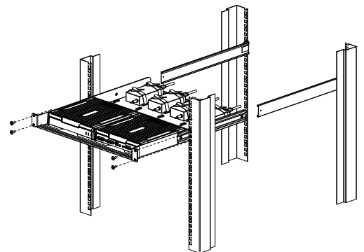
KE6948A 2-in-1U KE6948A 機架安裝套件 (2K-0013)
